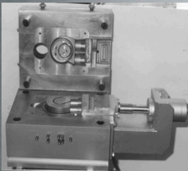
Matriz de inyección salida de gases calefactores.
