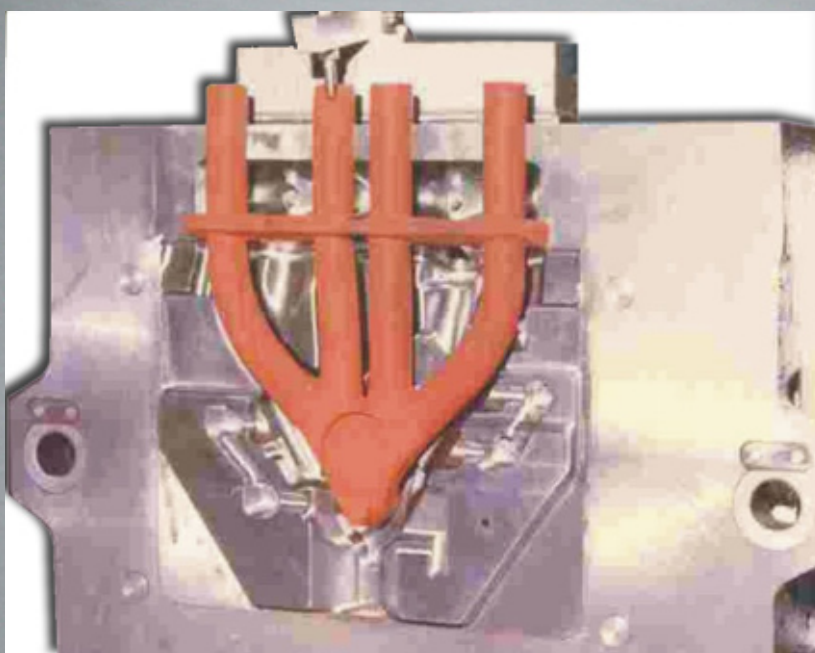
Coquilla múltiple admisión Volkswagen.
