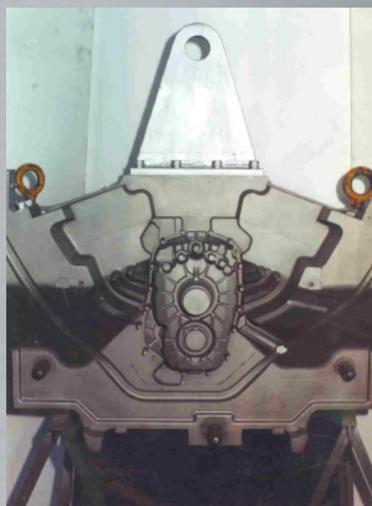
Coquilla tapa con anlajes caja de cambios ZF, cara fija con partes móviles y cara móvil
