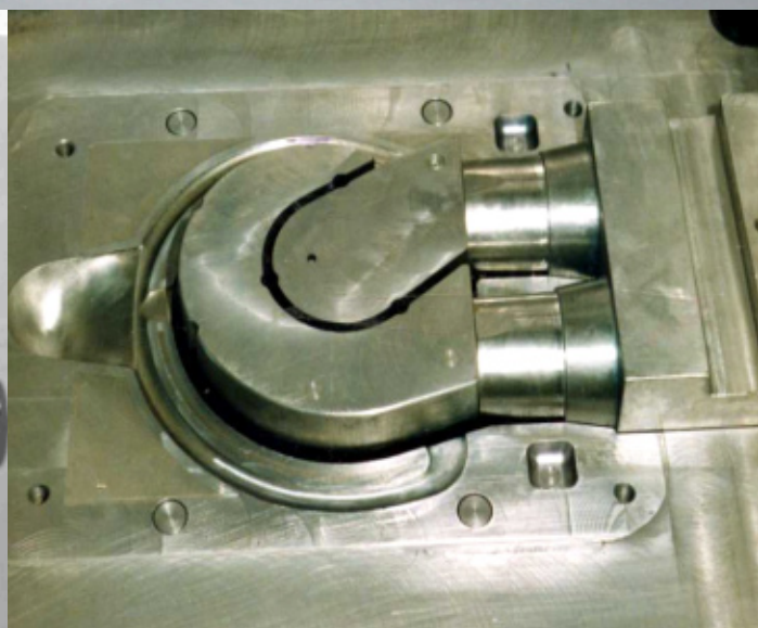
Matriz de inyección salida de gases calefactores.
