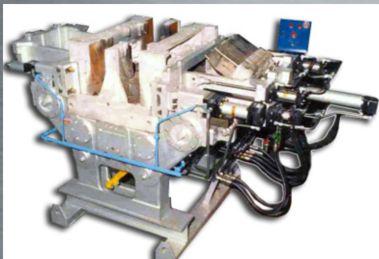
Coquilla y banco coquillero para tapa de cilindros Renault. Tres herramientas completos, con automatismos.
