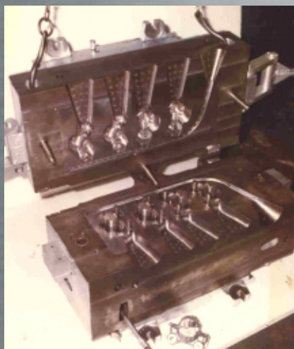
Coquilla caliper de Freno.
