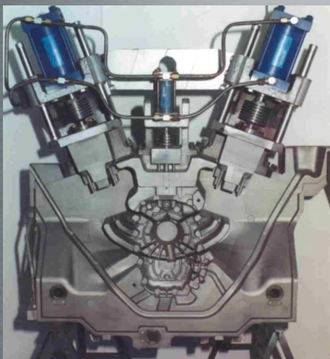
Coquilla tapa con anlajes caja de cambios ZF, cara fija con partes móviles y cara móvil
